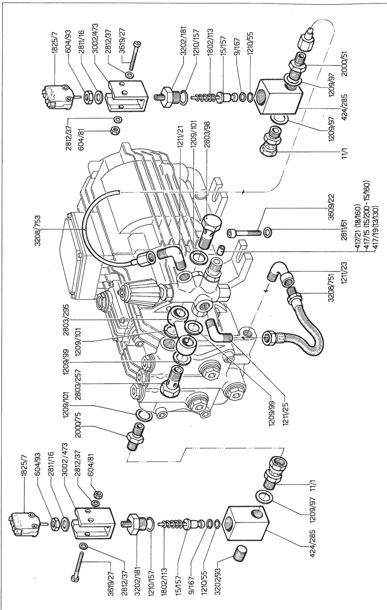
Raccordi collegamento
