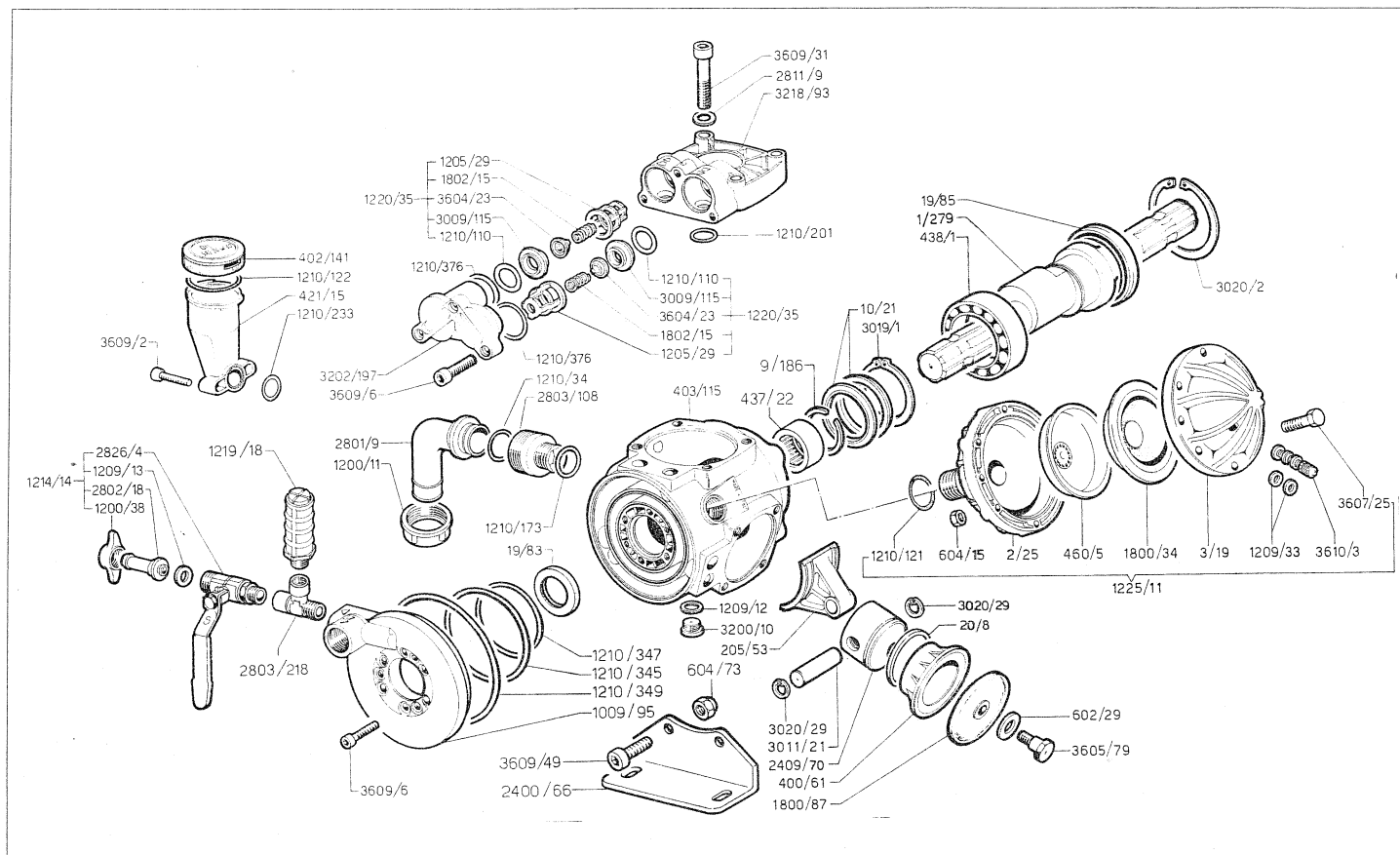
Albero passante 1" 3/8 M - 1" 3/8 M, con piedi (6078 0001 00)
