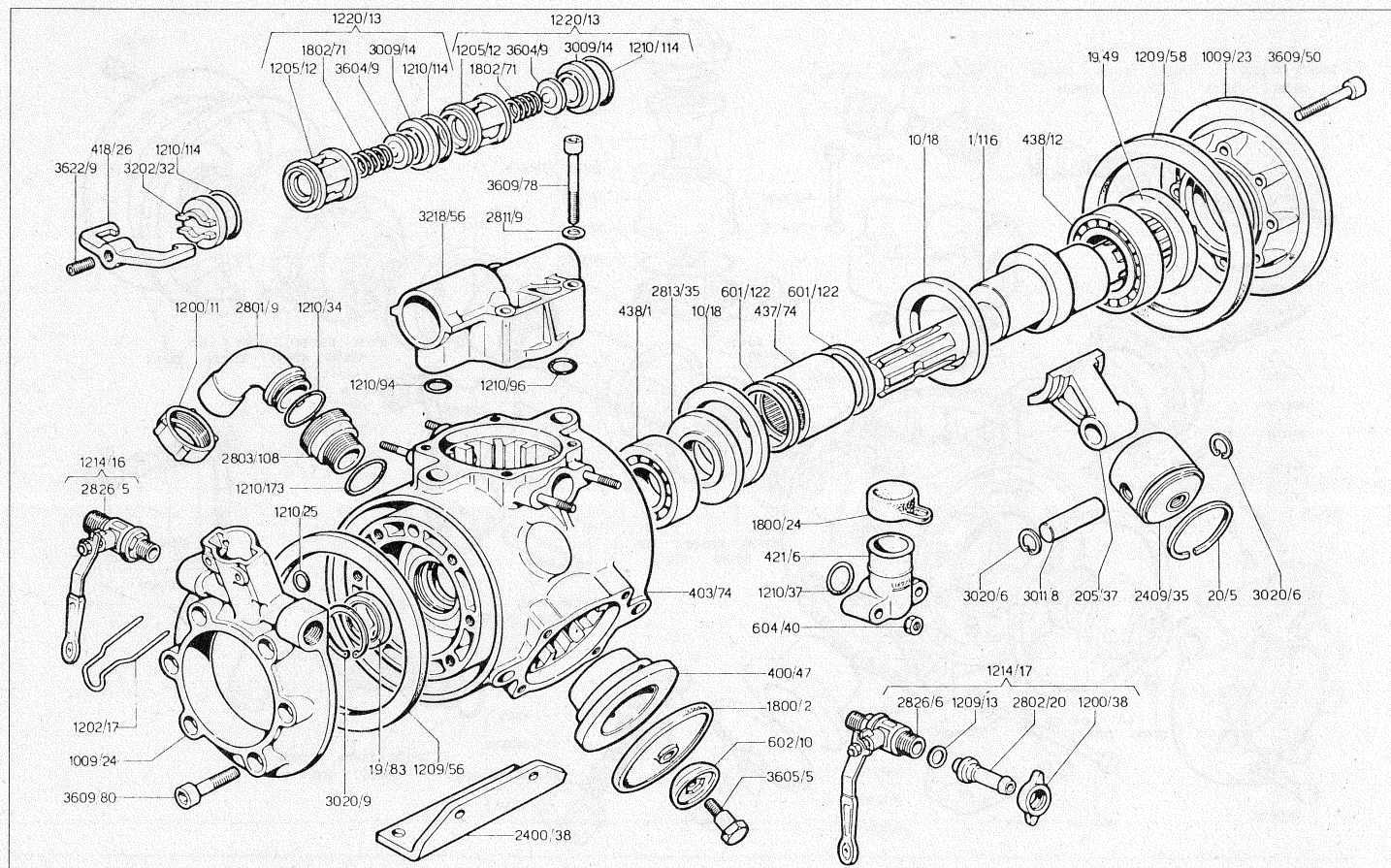
Albero passante 1" 3/8 M - 1" 3/8 M, con piedi (6054 0001 00)
