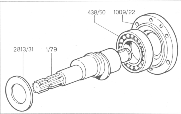
Varianti per albero passante 1" 3/8 M - cilindrico Ø 37 per riduttore R=1:1,5, con piedi (6036 0006 00)
