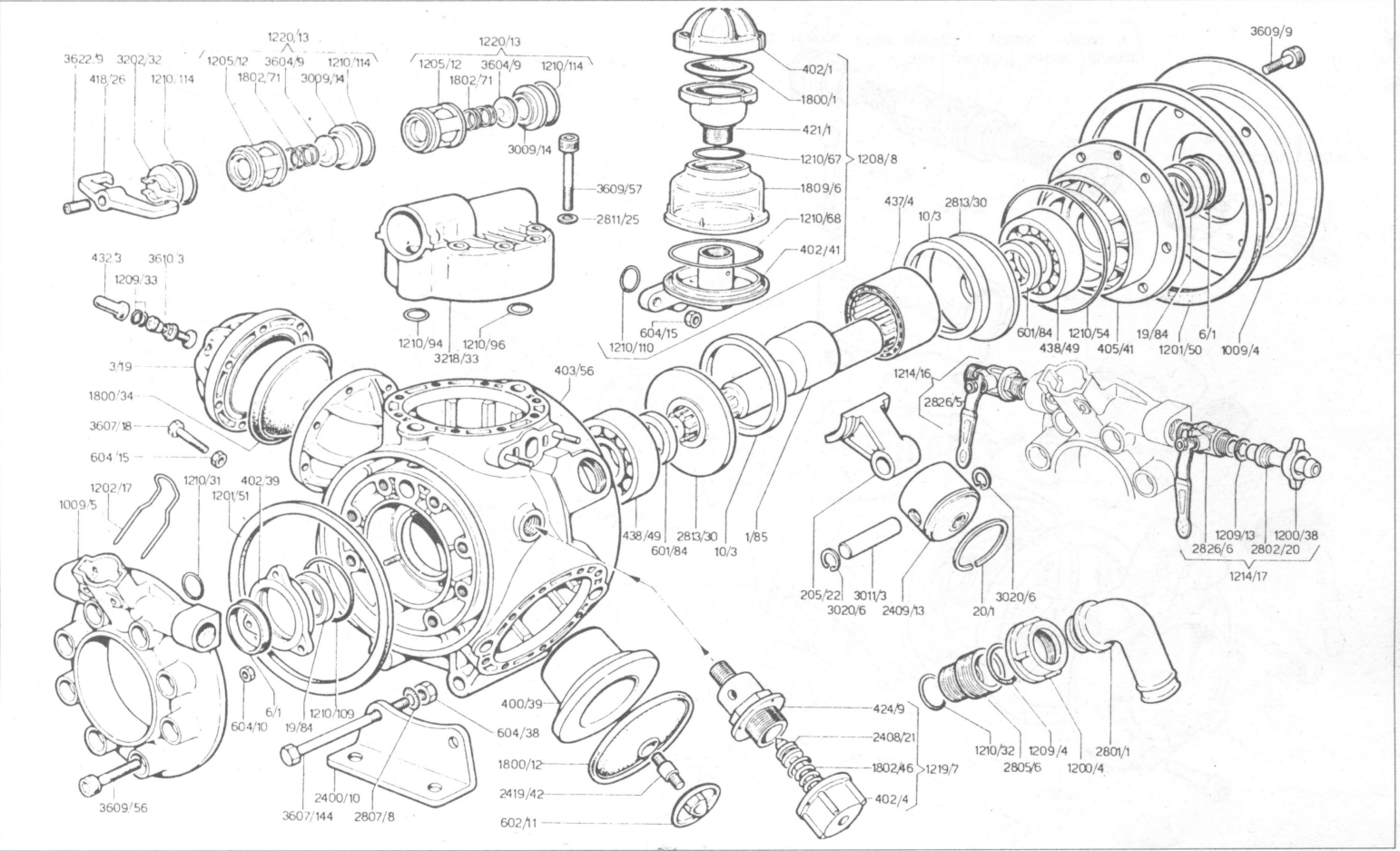
Albero passante 1" 3/8 M - 1" 3/8 M, con piedi (6036 0001 00)
