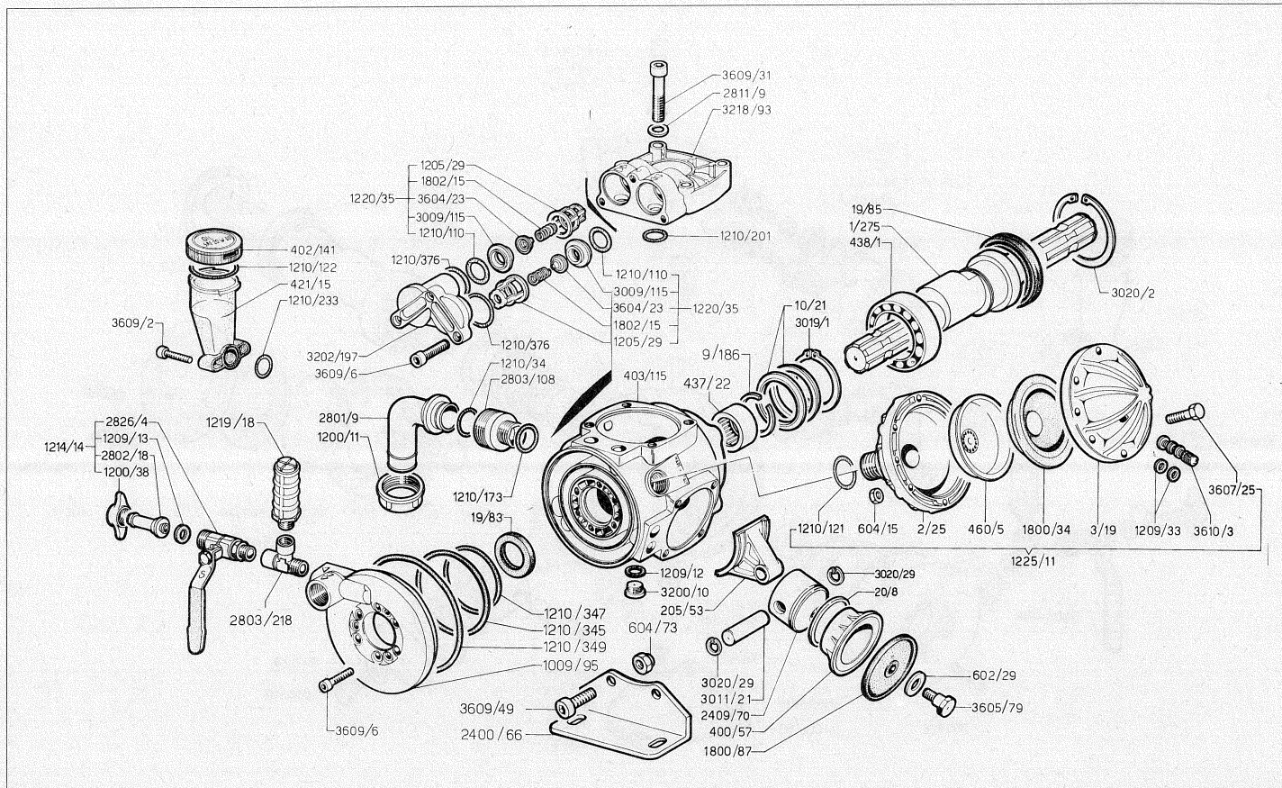
Albero passante 1" 3/8 M - 1" 3/8 M, con piedi (6076 0001 00)
