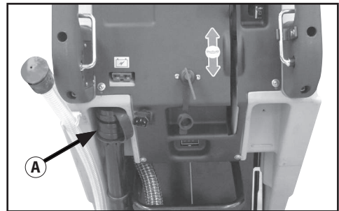
Foto 25 A) Schlauch zum Entleeren des Sammelbehälters mit einstellbarem Fluss
